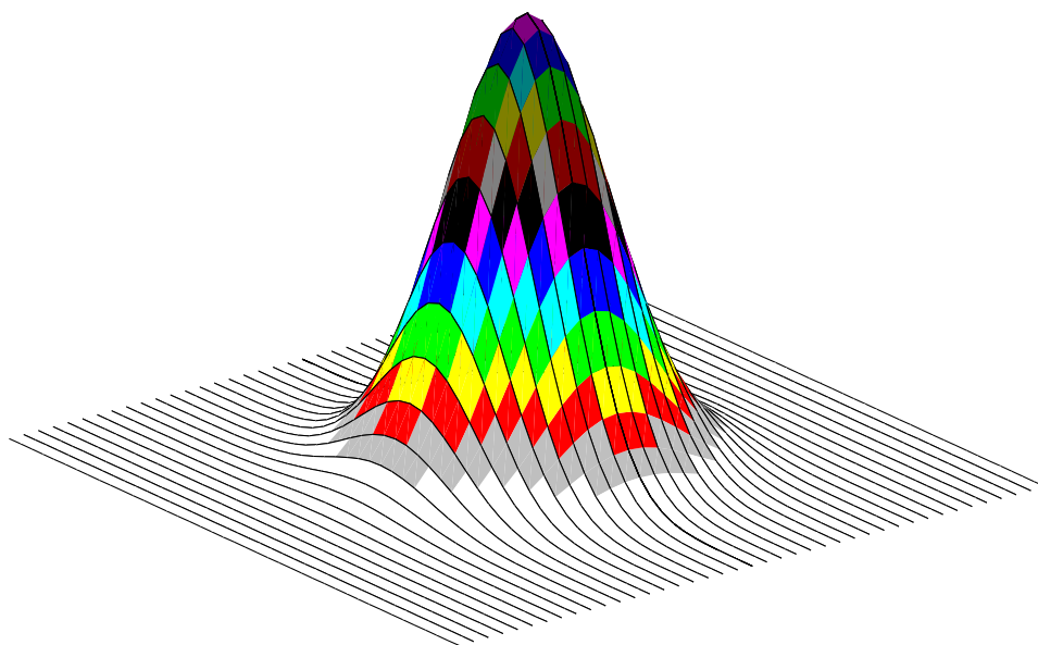
Obr. 1: Fundamentální řešení operátoru vedení tepla v \mathbf{E}^{2+1} ve fixovaném čase t = 0.1 .
