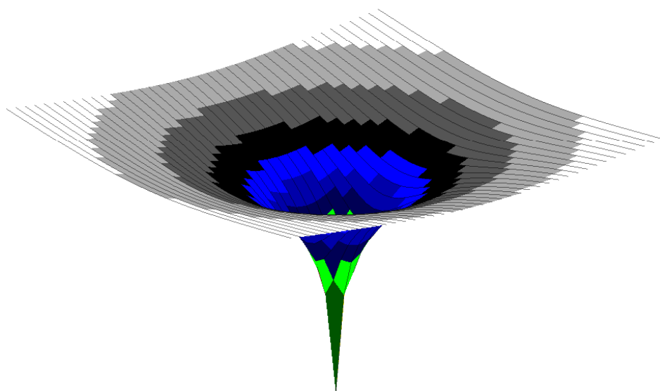
Obr. 3: Fundamentální řešení Laplaceova operátoru v E^2 .
