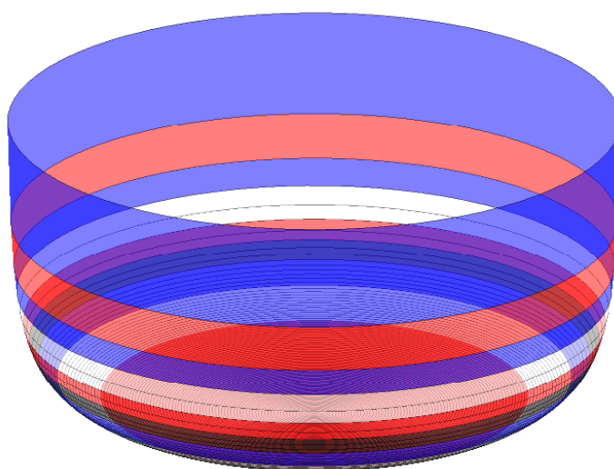
Obr. 2: Fundamentální řešení vlnového operátoru v \mathbf{E}^{2+1} ve fixovaném čase .
